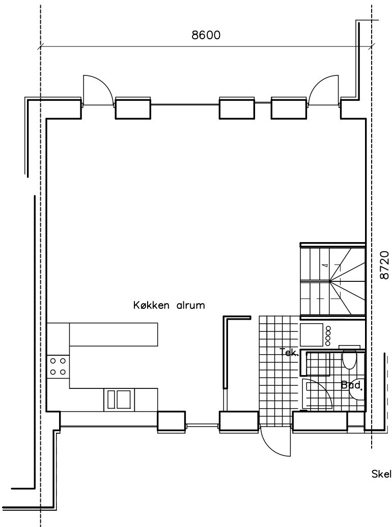
Stueplan
