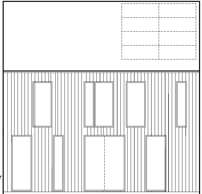
Facade syd/øst
