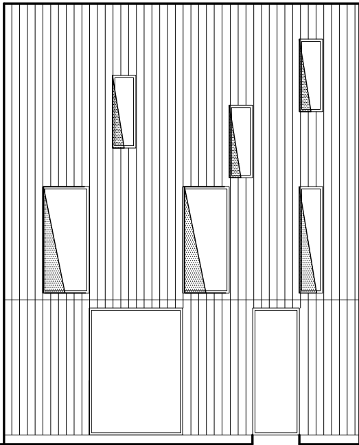
Facade nord/vest
